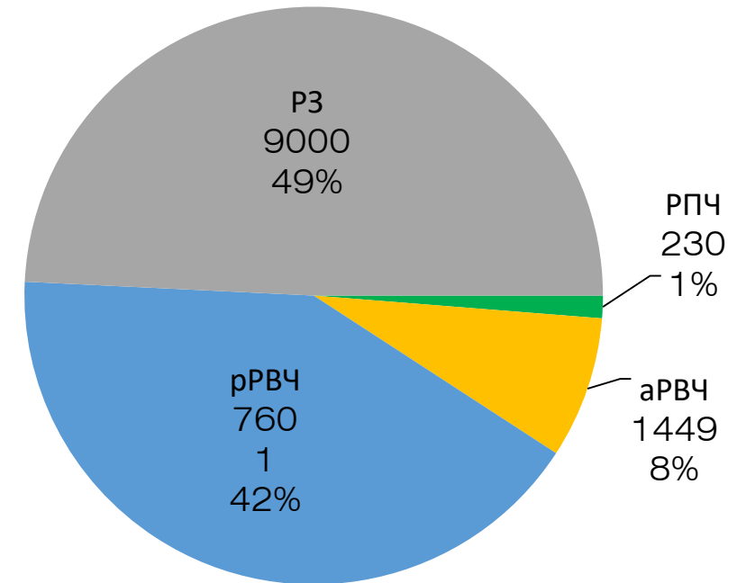
ДП із регулювання частоти та потужності в ОЕС України, МВт
