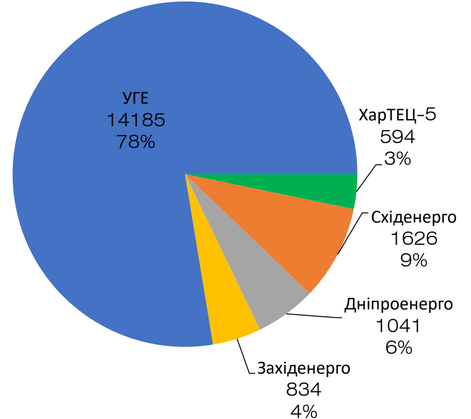
ОЕС України, МВт
